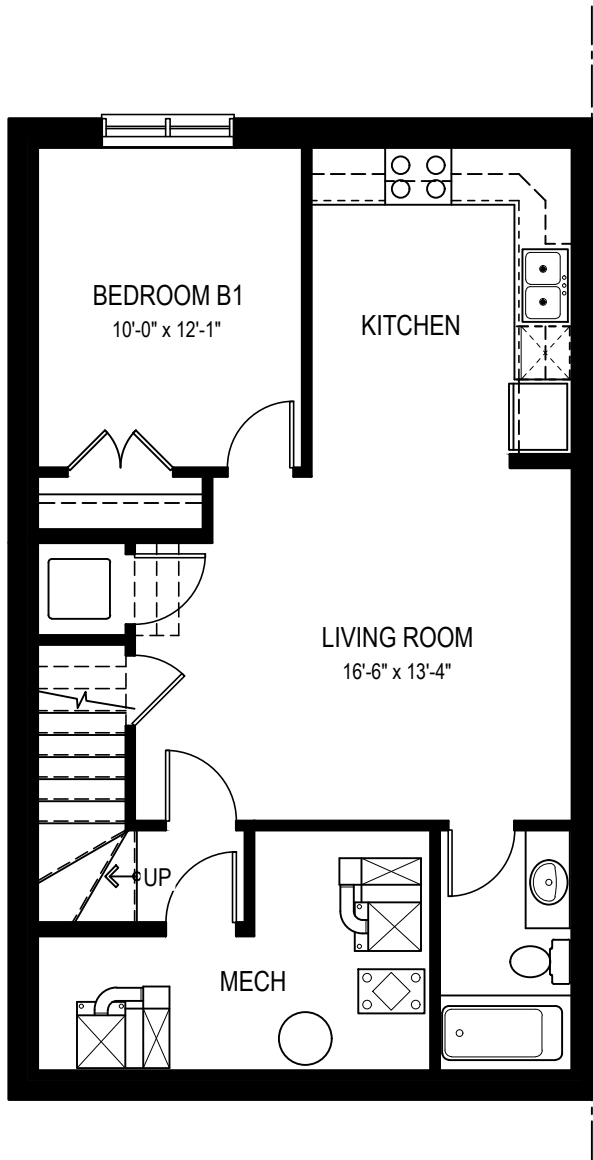
BASEMENT SUITE OPTION 596 sq.ft.
